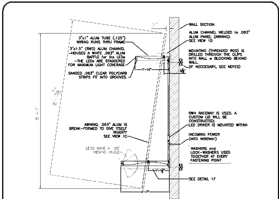
1 SIDE / SECTION B SCALE: 1/2"=1'-0"
