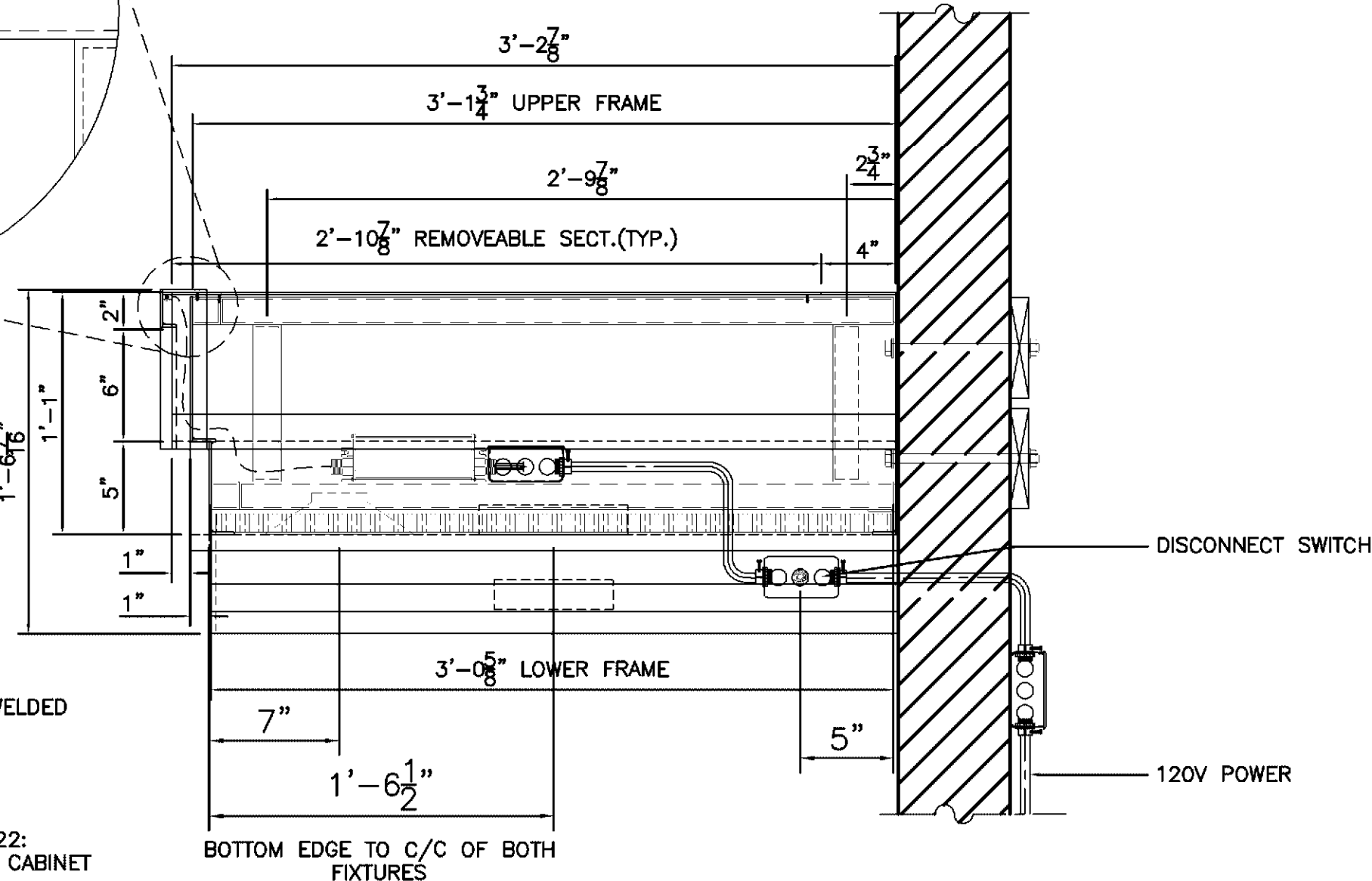
VIEW 1C: END SCALE: 1-1/2"=1'
