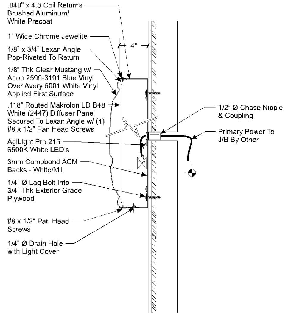
CROSS SECTION SCALE: 1 1/2" = 1'-0"
