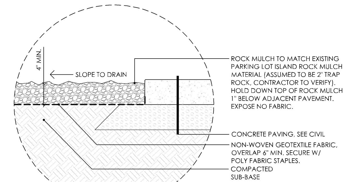
1 rock mulch typ. scale: 1" = 1'-0"
